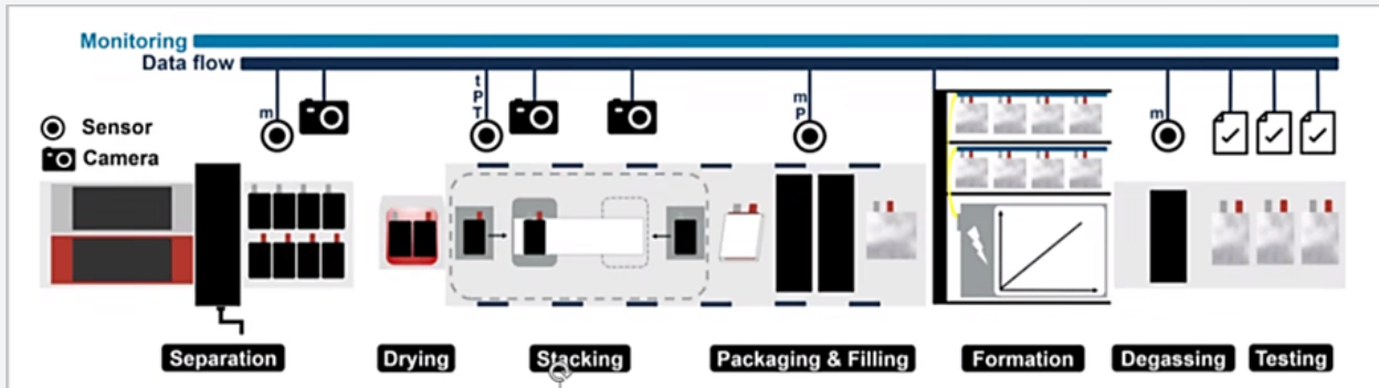
Abb. 1 Schematischer Ablauf der Batteriezellproduktion.
