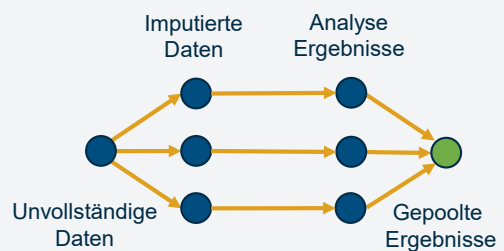
Abb. 7 Imputation durch Rekonstruktion aus teilweise unvollständigen Datensätzen.
