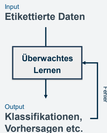
Abb. 8 Überwachtes Lernen.
