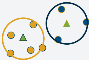
Abb. 5 Imputation aus ähnlichen Datensätzen.
