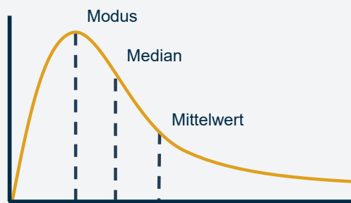
Abb. 3 Imputation durch Schätzung aus Lageparametern.
