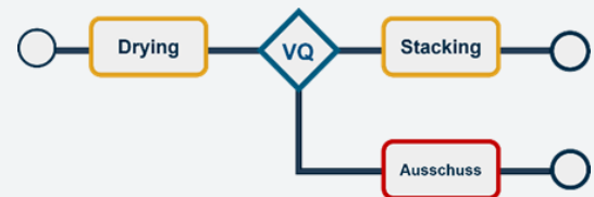
Abb. 14 Vereinfachtes Prozessschaubild mit Virtual Quality Gate.
